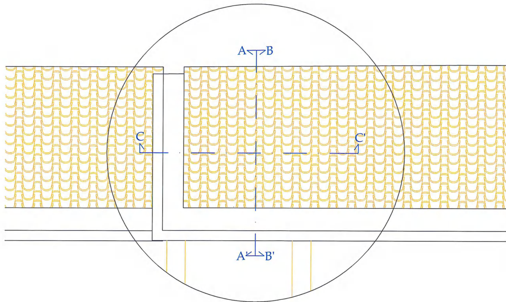
PIANTA COPERTURA
