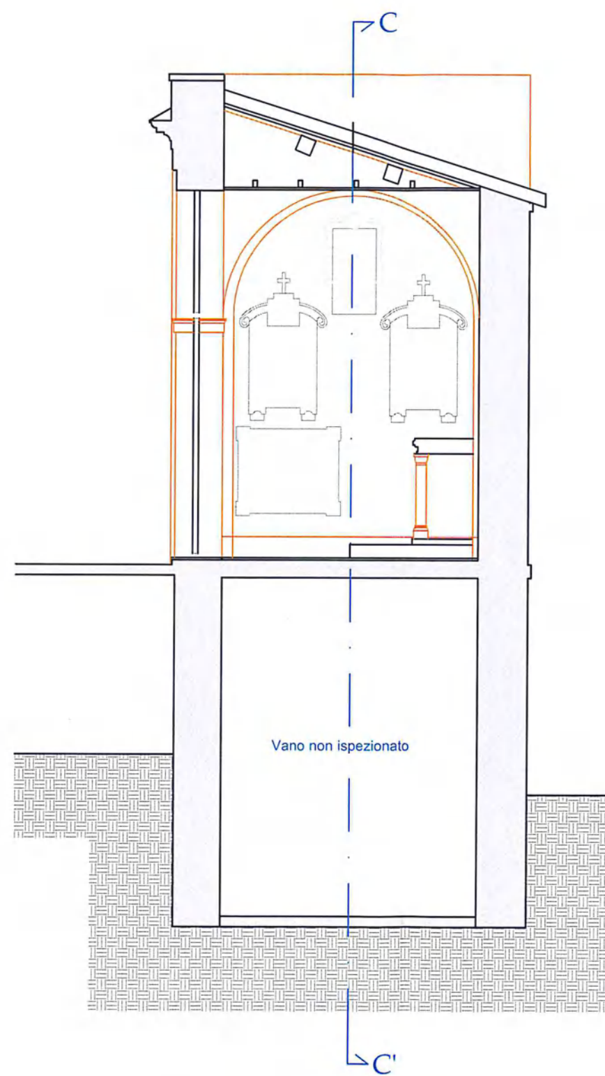
SEZIONE A-A'
