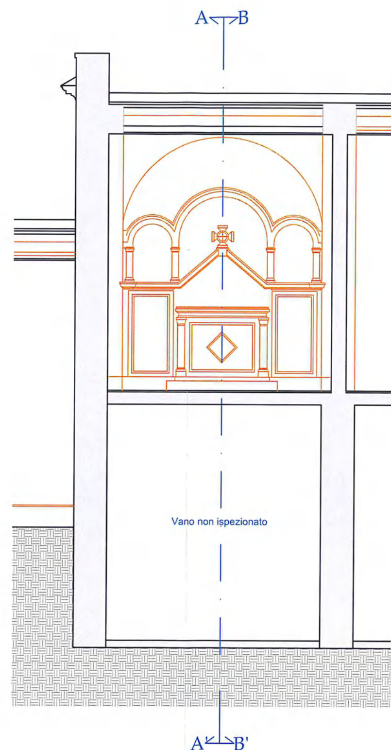
SEZIONE C-C'
